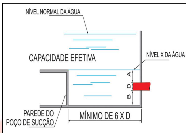
Figura B.2: Tomada lateral de sucção para bomba principal
