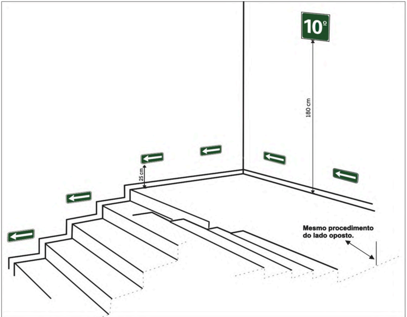
Figura C-8: Sinalização complementar. Exemplo de rodapé
