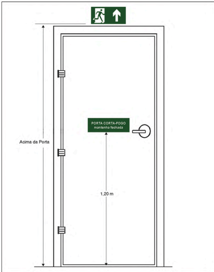
Figura C-1: Sinalização de porta corta-fogo (vista do hall)
