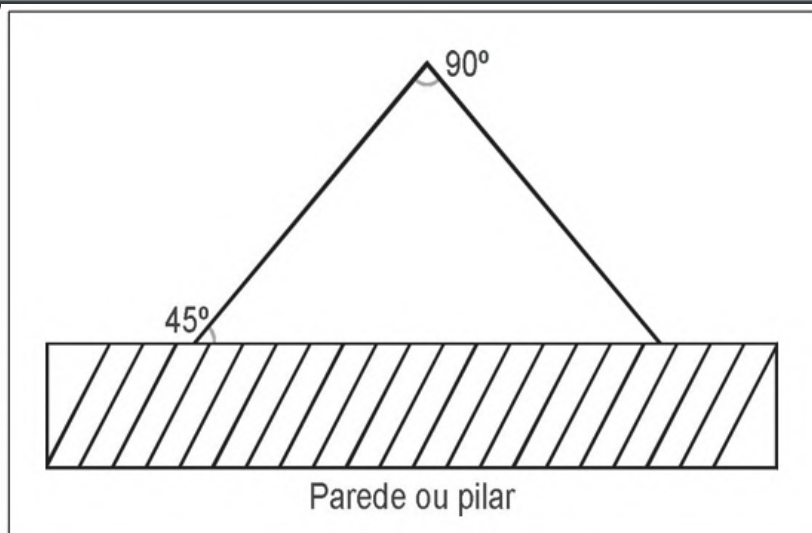
Figura 1: Instalação de placa angular
