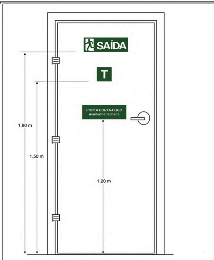
Figura C-3: Sinalização de porta corta-fogo (vista da escada)
