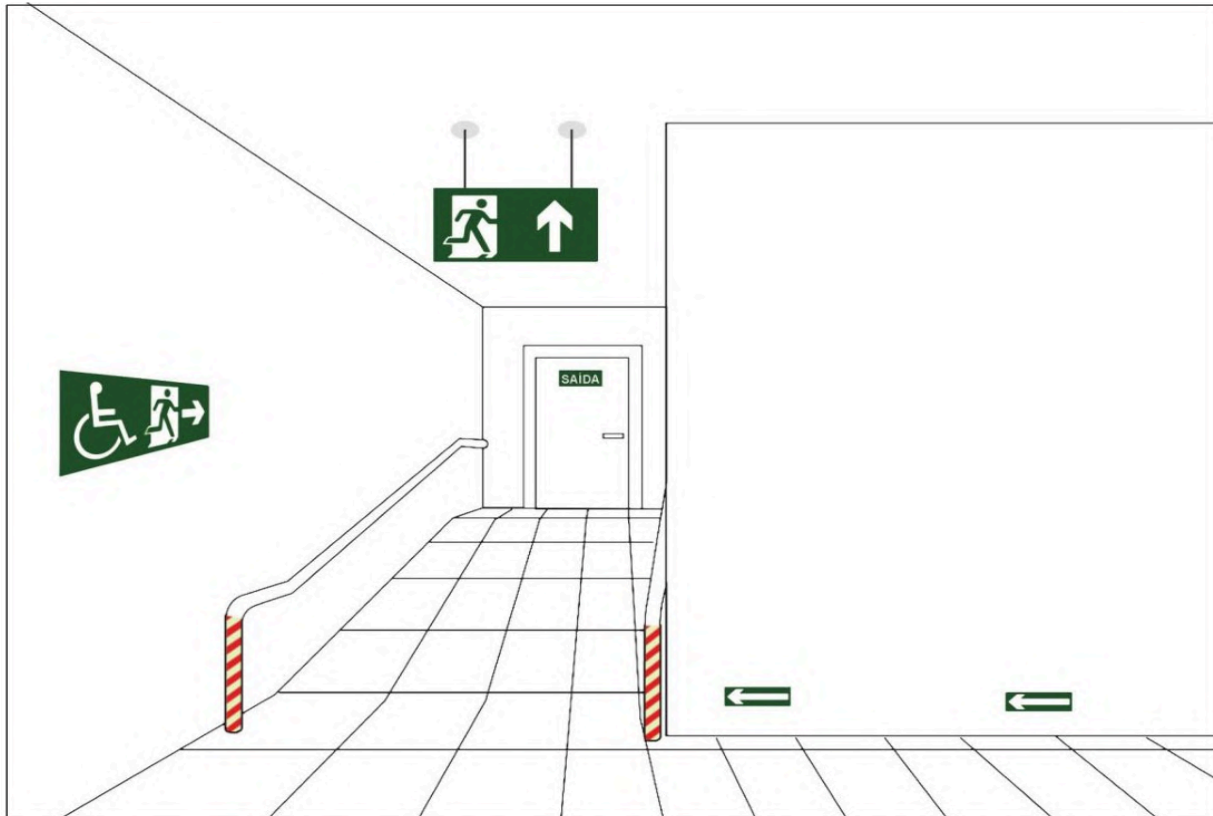
Figura C-15: Sinalização de saída em rampa.
