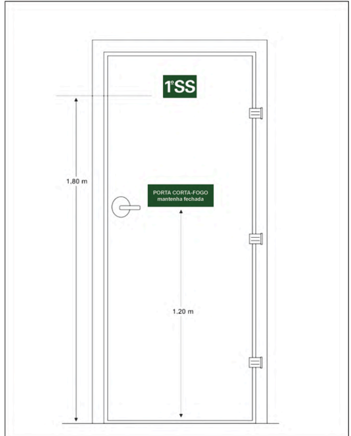
Figura C-2: Sinalização de porta corta-fogo (vista da escada)
